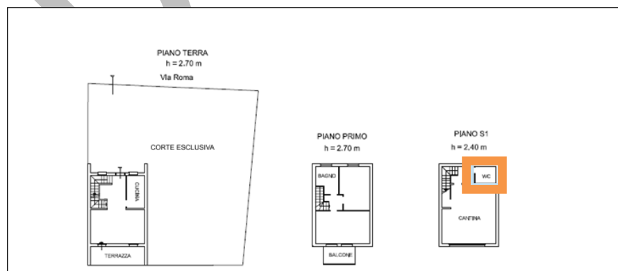
Figura 3.43: esempio di locale accessorio a servizio diretto di locali indiretti comunicanti (poligono tipo B)
